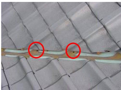
谷板金腐食による穴
