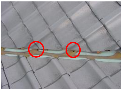
谷板金腐食による穴
